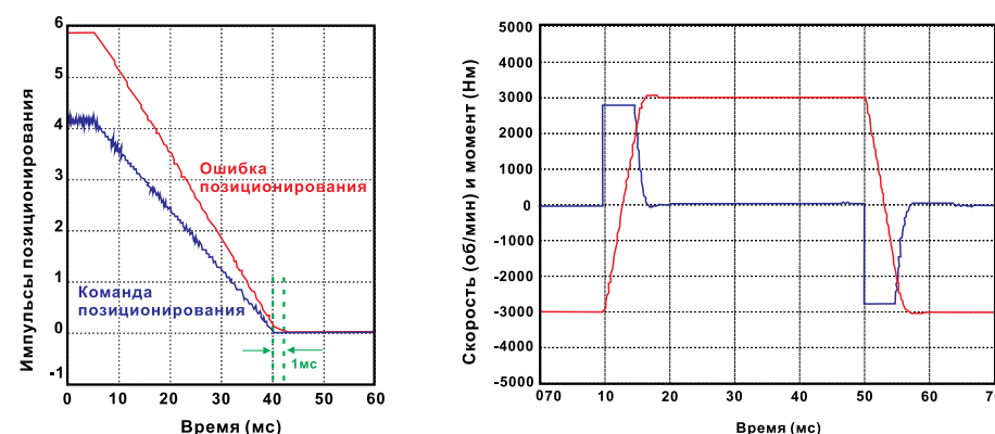
Графики для серводвигателя с фланцем 60мм, мощностью 400Вт
